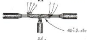
3.6 การต่อสายเมนแบบ (Ordinary Tape Splice)
