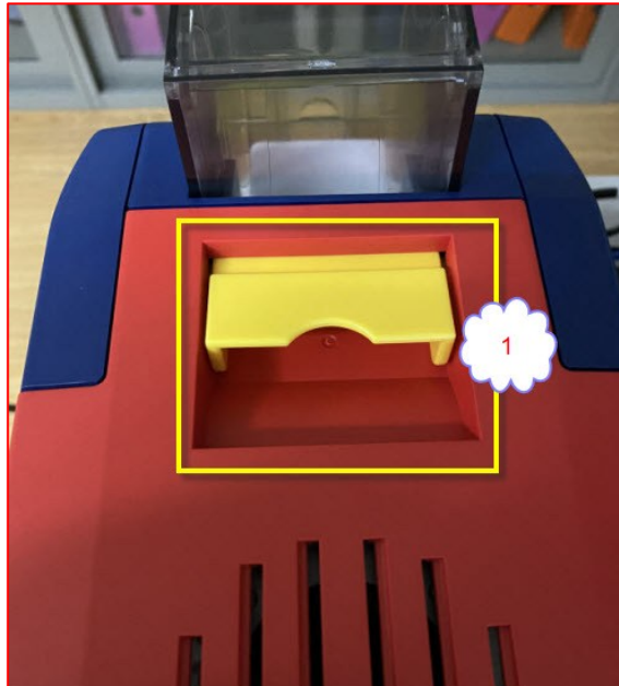
(1) เปิดฝาช่องใส่ Ribbon ด้านบนเครื่องพิมพ์บัตร โดยยกตัวล็อกสีเหลืองขึ้น
