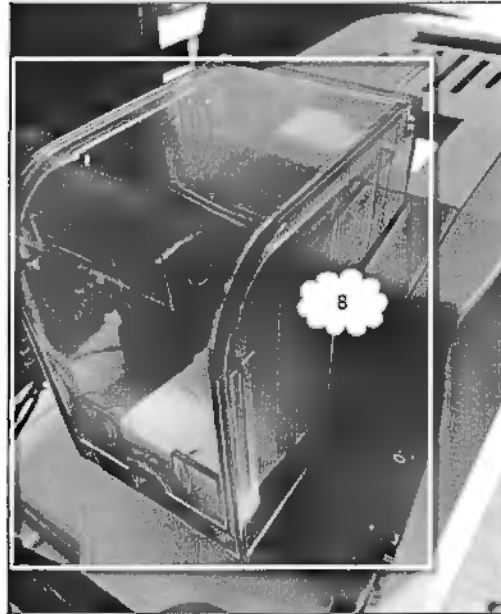
(8) นำถาดป้อนบัตรพลาสติกมาประกอบที่ด้านหลังเครื่องพิมพ์บัตรพลาสติก
