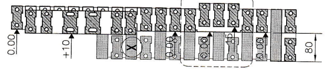
รูปตัด 1-1 ขนาดชั้น 1:10
